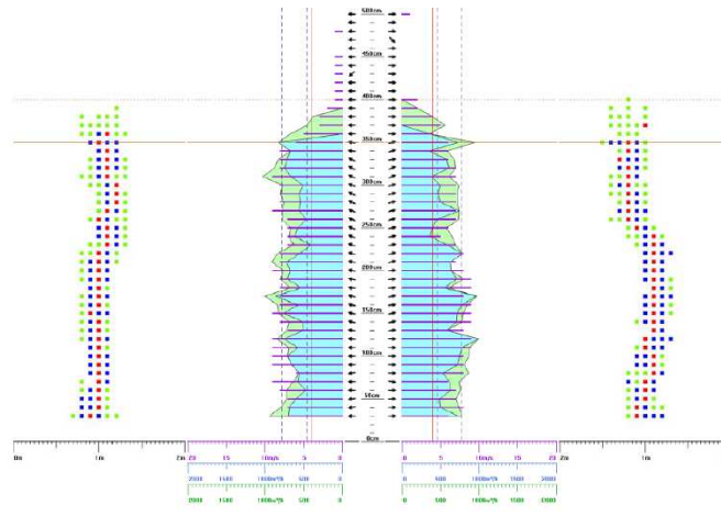
Messprotokoll - Gebläseluftverteilung - Sollverteilung
